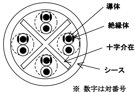
付図1 構造図
